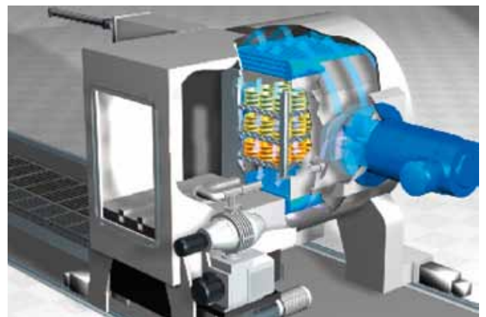
Shuttlemodul bestehend aus Transport- und Abschreckkammer
